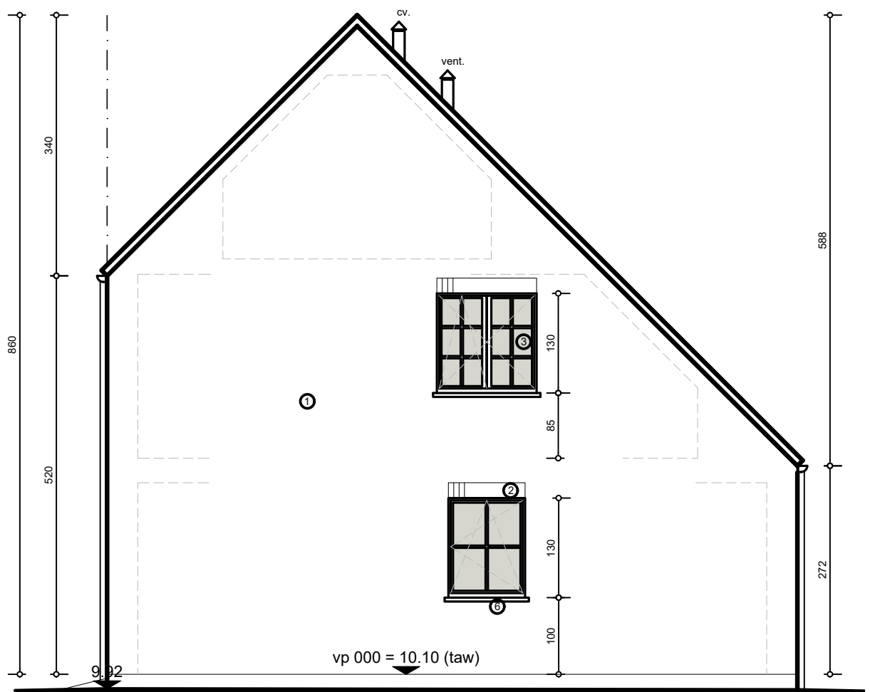
ZIJGEVEL RECHTS (met terreinprofiel)
