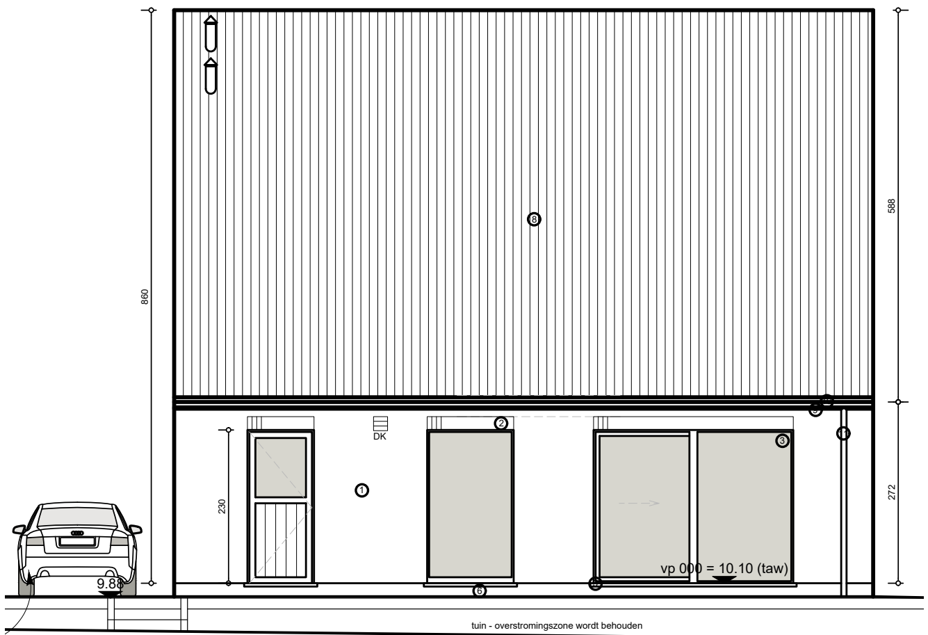
ACHTERGEVEL (met terreinprofiel)
